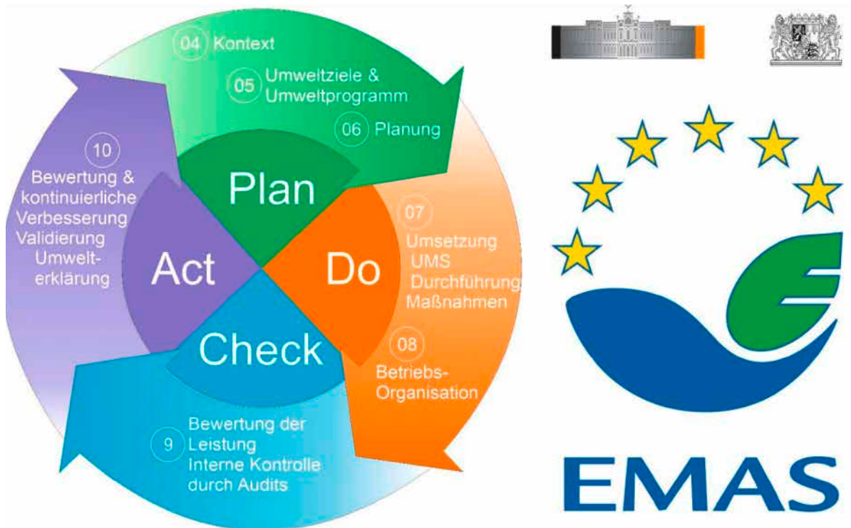
Abbildung 2: Plan-Do-Check-Act-Zyklus 1
